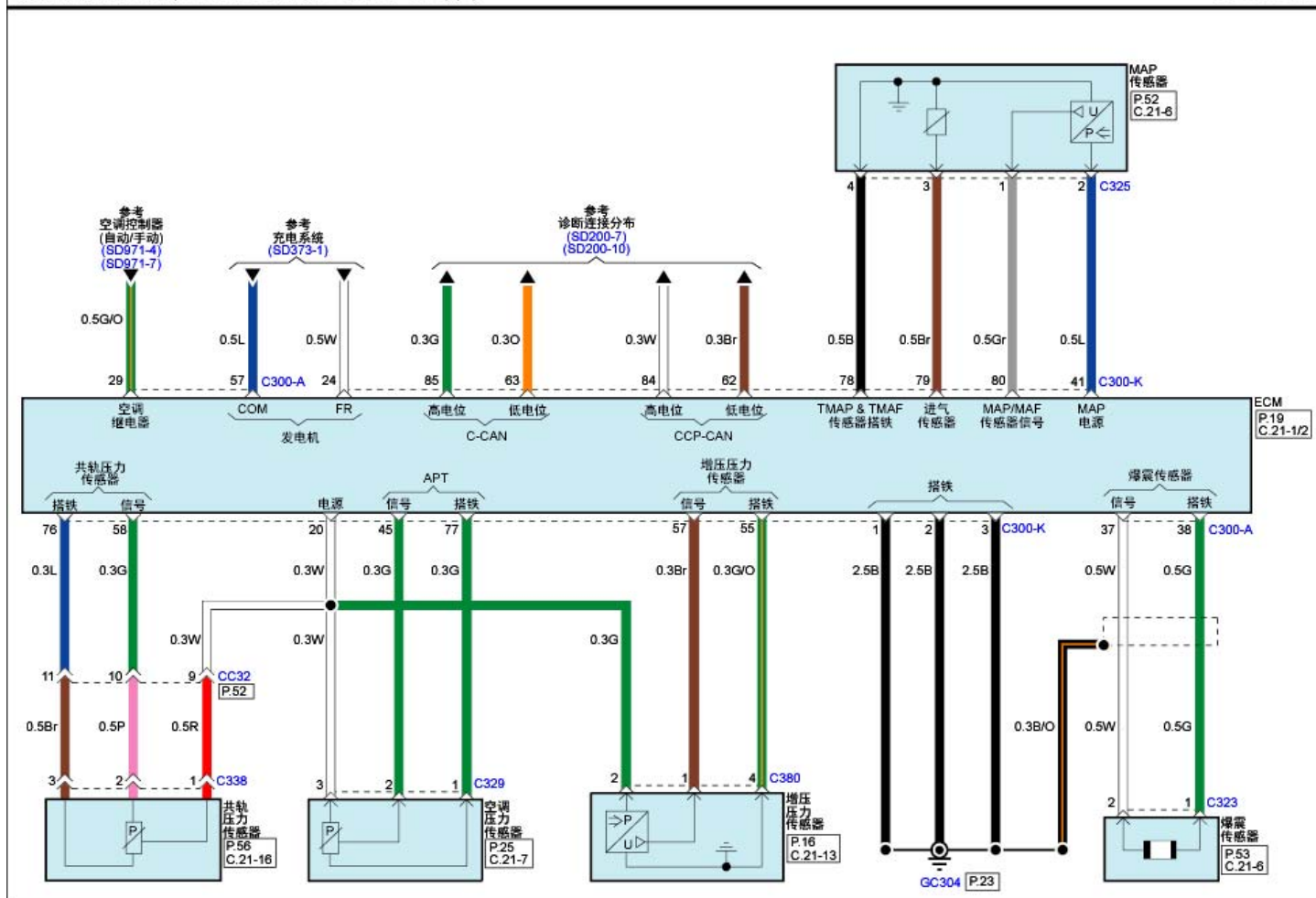
发动机控制系统(G4FJ : GAMMA 1.6L T-GDI)(7)
